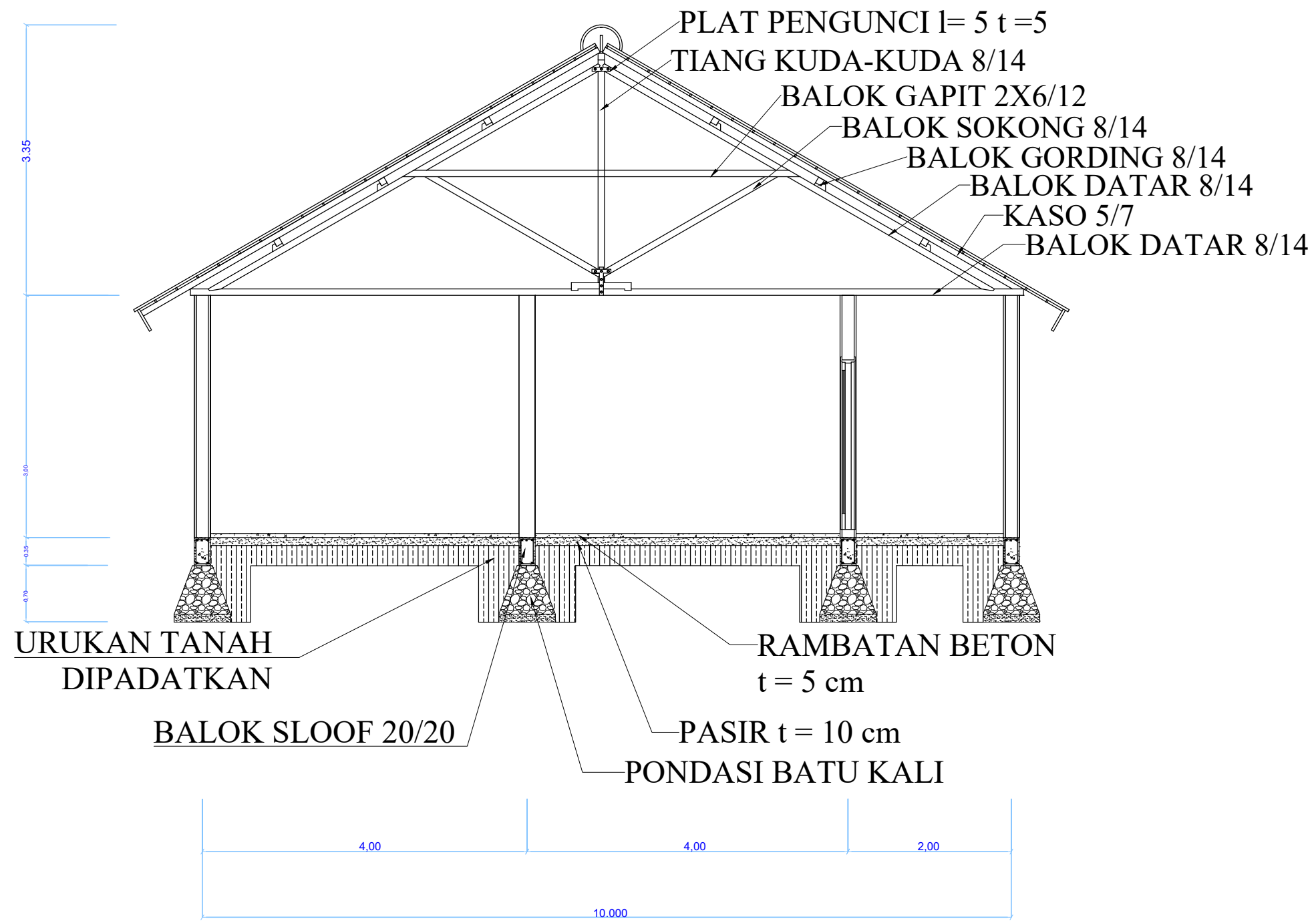
POTONGAN S-02
