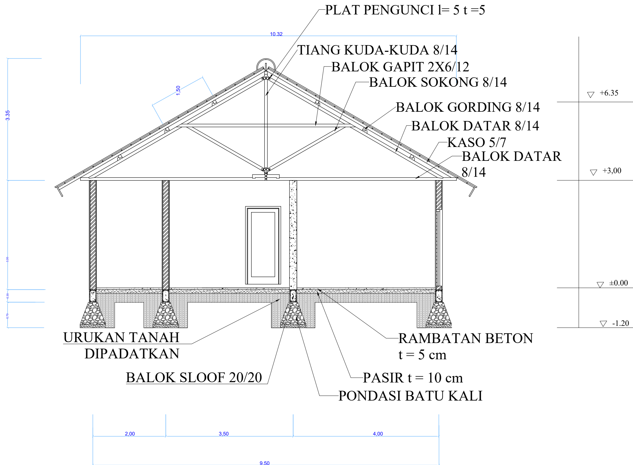
POTONGAN S-01
