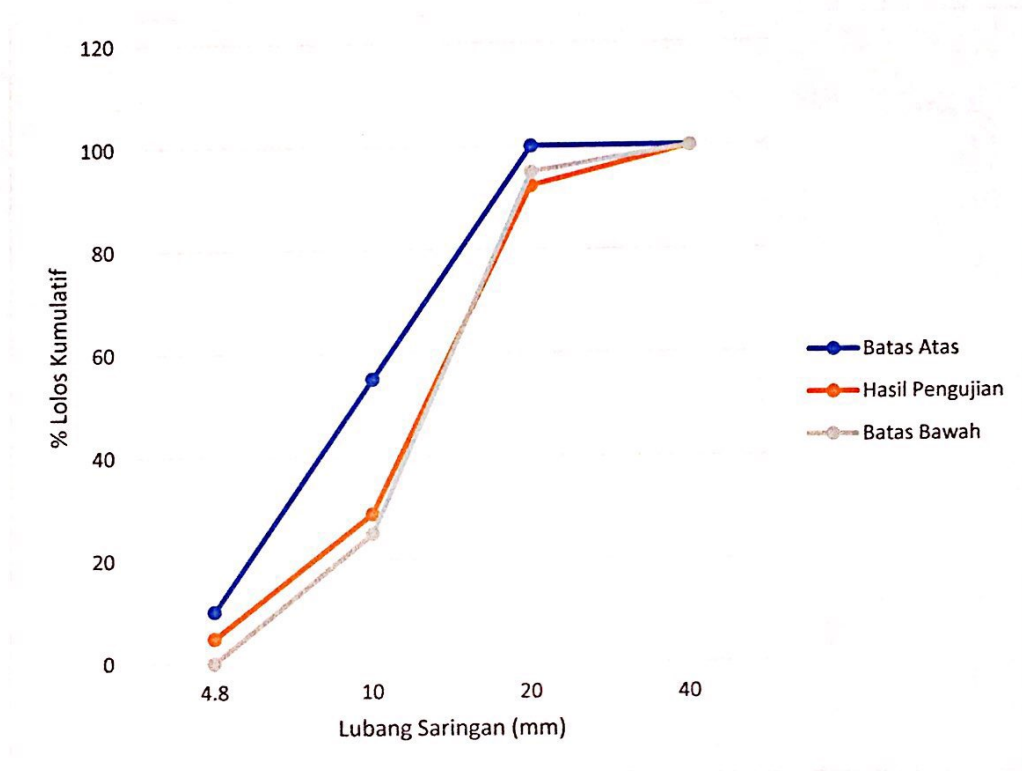
GAMBAR ANALISA SARINGAN AGREGAT KASAR
