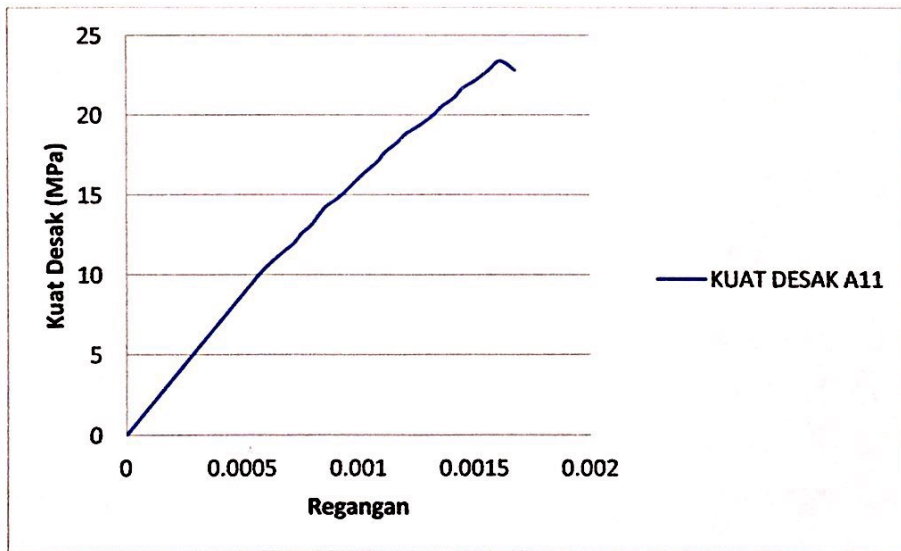
Gambar L11-2 Koreksi Kuat Desak Beton A11
