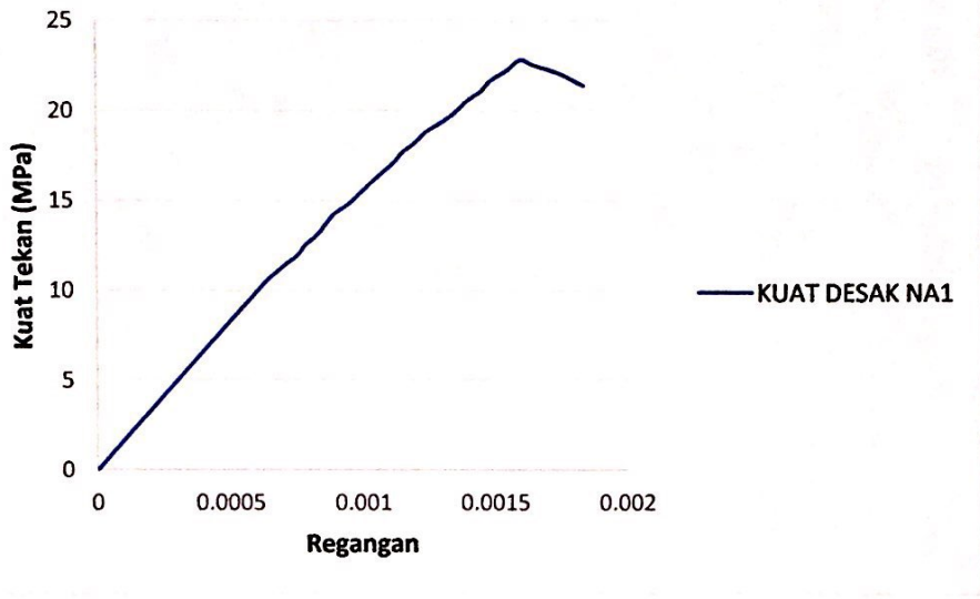
Gambar L11-1 Koreksi Kuat Desak Beton NA1
