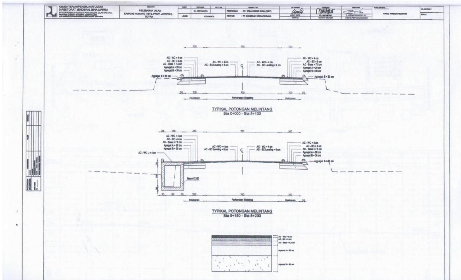
Gambar L4.1 Potongan Melintang Jalan
