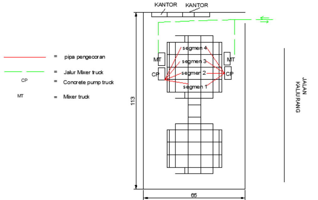
Gambar L 4.1 Skema Pergerakan Alat Berat Dengan Kondisi Real di Lapangan
