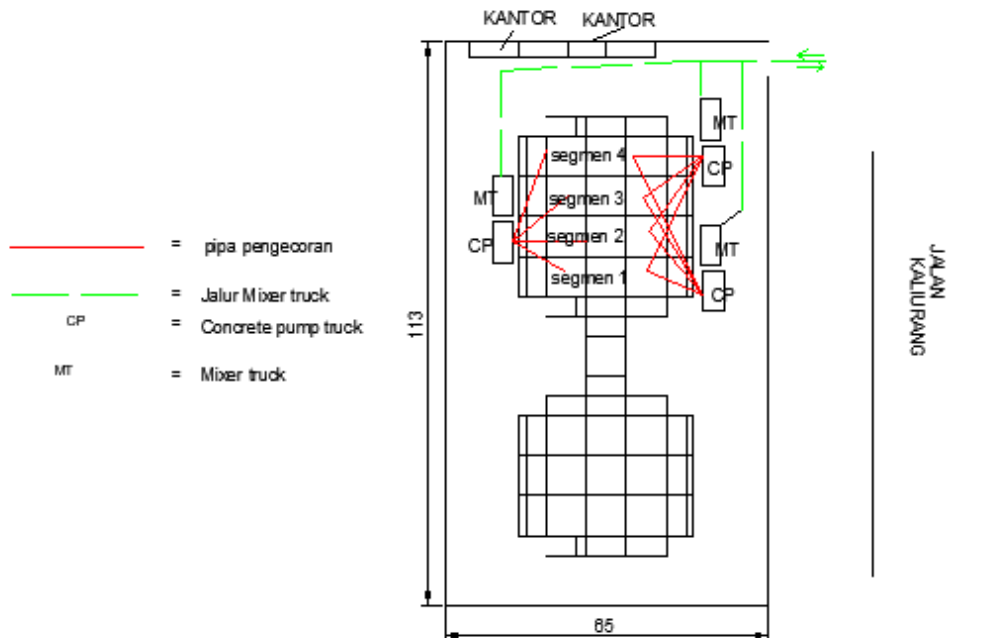
Gambar L 4.3 Skema Pergerakan Alat Berat Pada Alternatif 2
