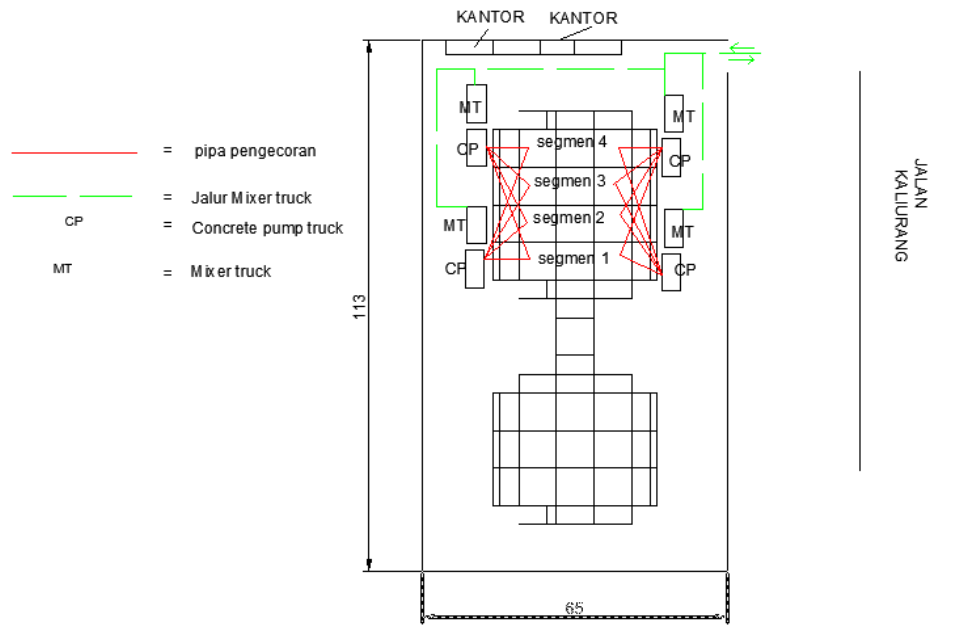
Gambar L 4.4 Skema Pergerakan Alat Berat Pada Alternatif 3
