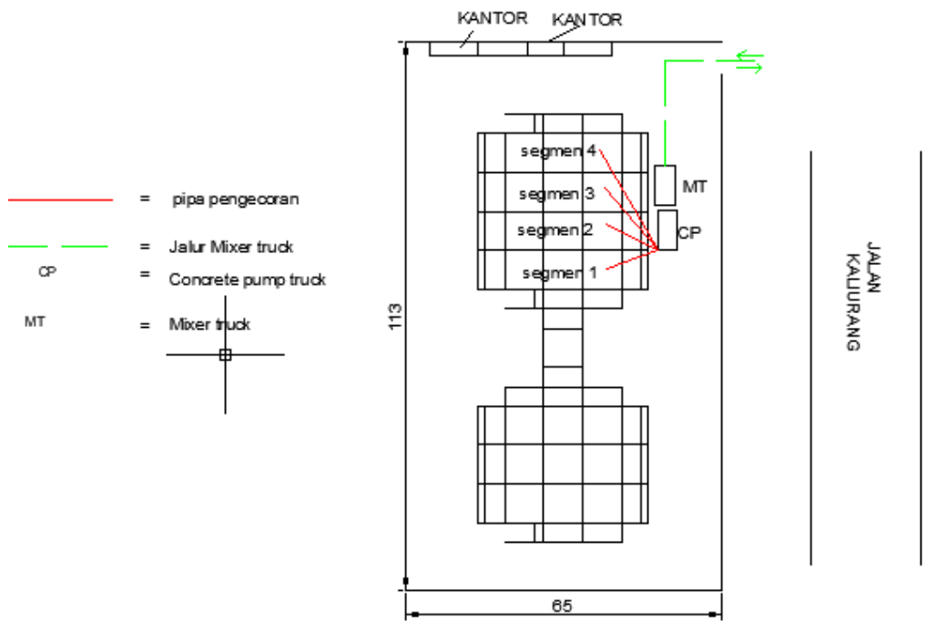
Gambar L 4.2 Skema Pergerakan Alat Berat Pada Alternatif 1
