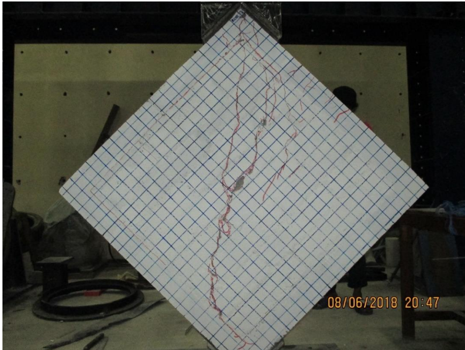
Gambar L-5.1 Benda Uji Reinforced Concrete Infill Masonry Wall 3 Setelah Diuji
