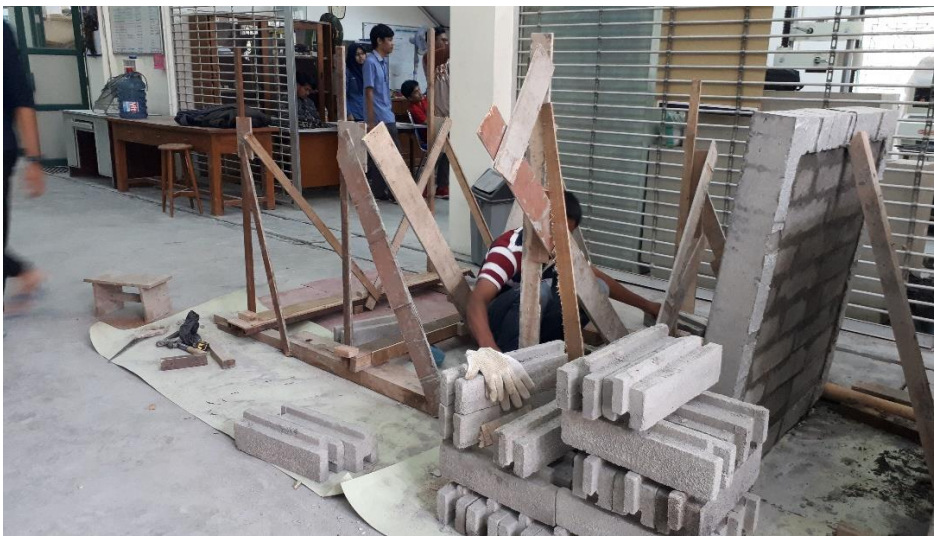
Gambar L-3.10 Proses Pembuatan Bekisting Dinding Tanpa Perkuatan
