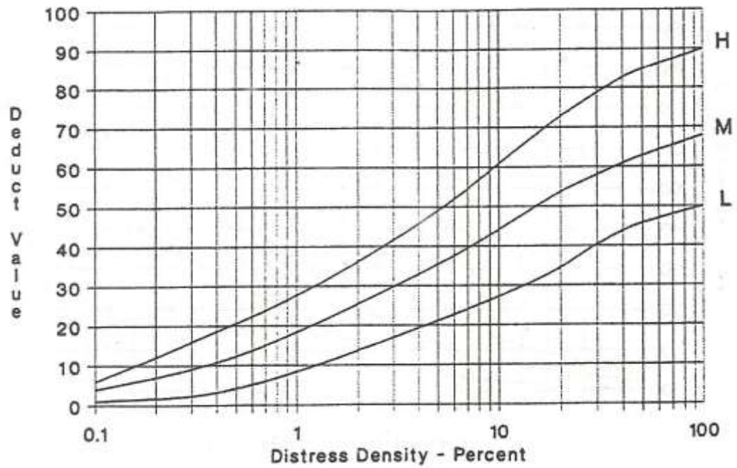
Alur ( Ruts )
