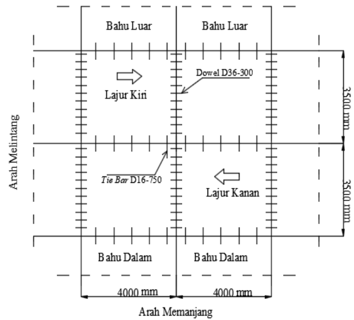
Penulangan Sambungan Metode Bina Marga 2017
