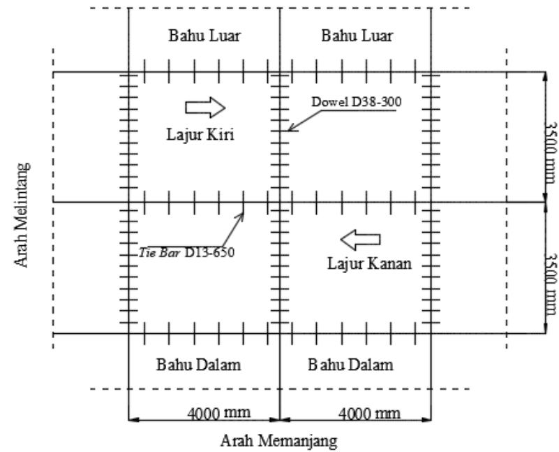
Penulangan Sambungan Metode AASHTO 1993
