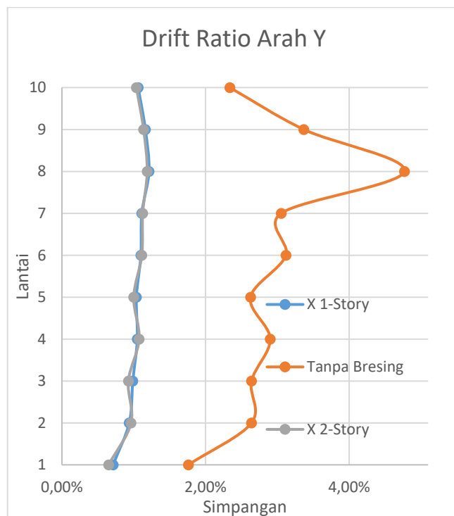
Gambar L-4.6 Hubungan Drift Ratio Arah Y
