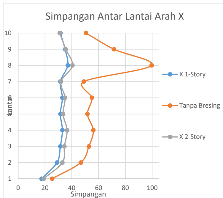
Gambar L-4.3 Simpangan Antar Lantai Arah X
