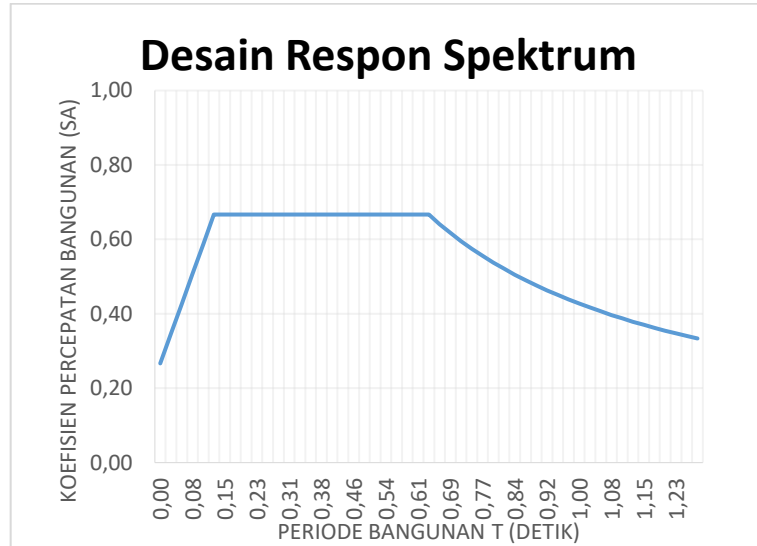
Gambar L-4.1 Desain Respon Spektrum
