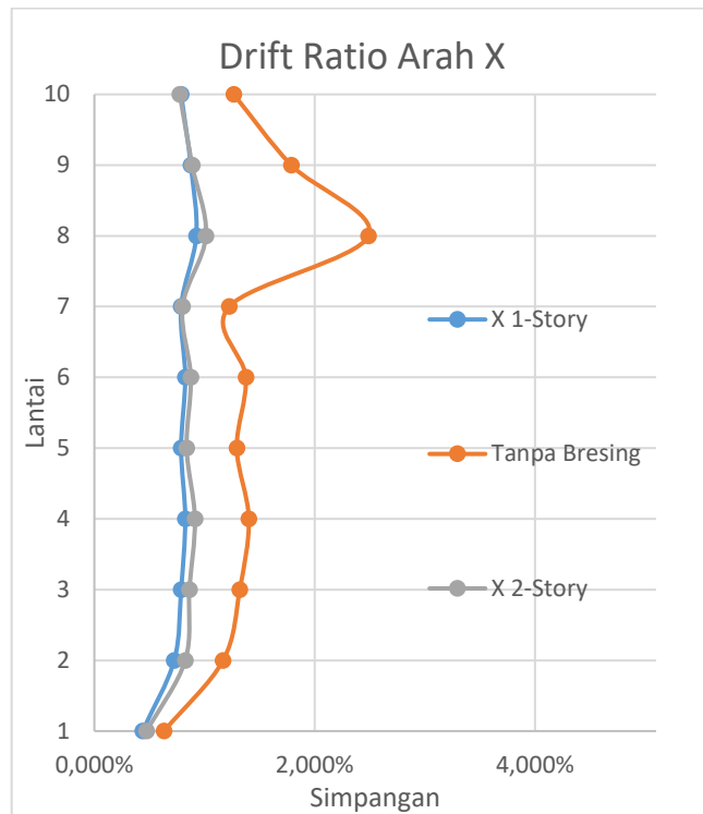
Gambar L-4.5 Hubungan Drift Ratio Arah X
