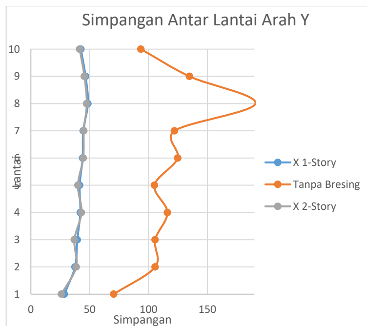
Gambar L-4.4 Simpangan Antar Lantai Arah Y
