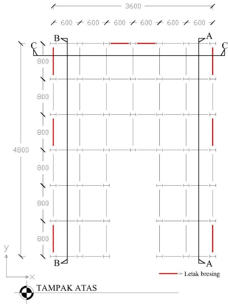
Gambar L-1.1 Pemodelan Denah Bangunan Tampak Atas
