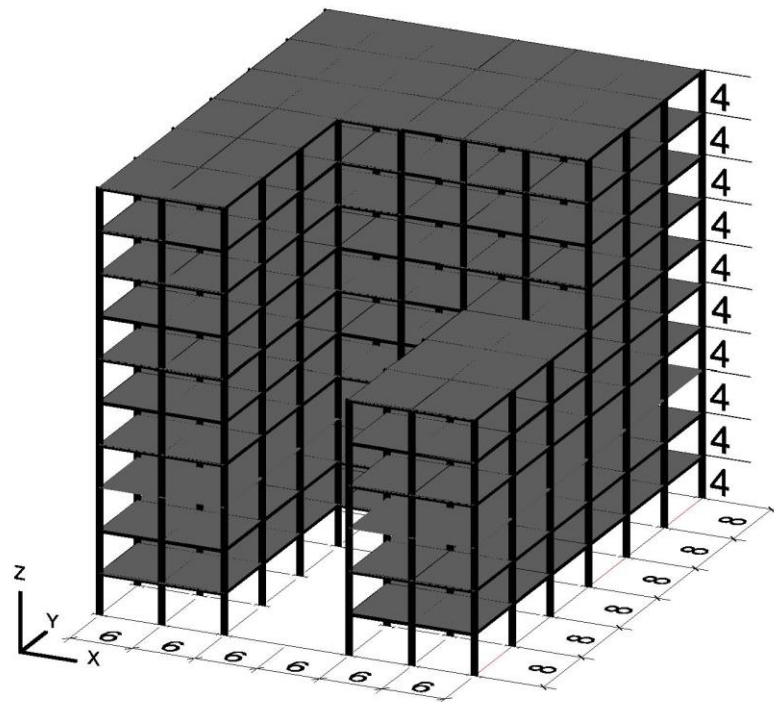
Gambar L-1.2 Pemodelan 3D Bangunan Tanpa Bresing
