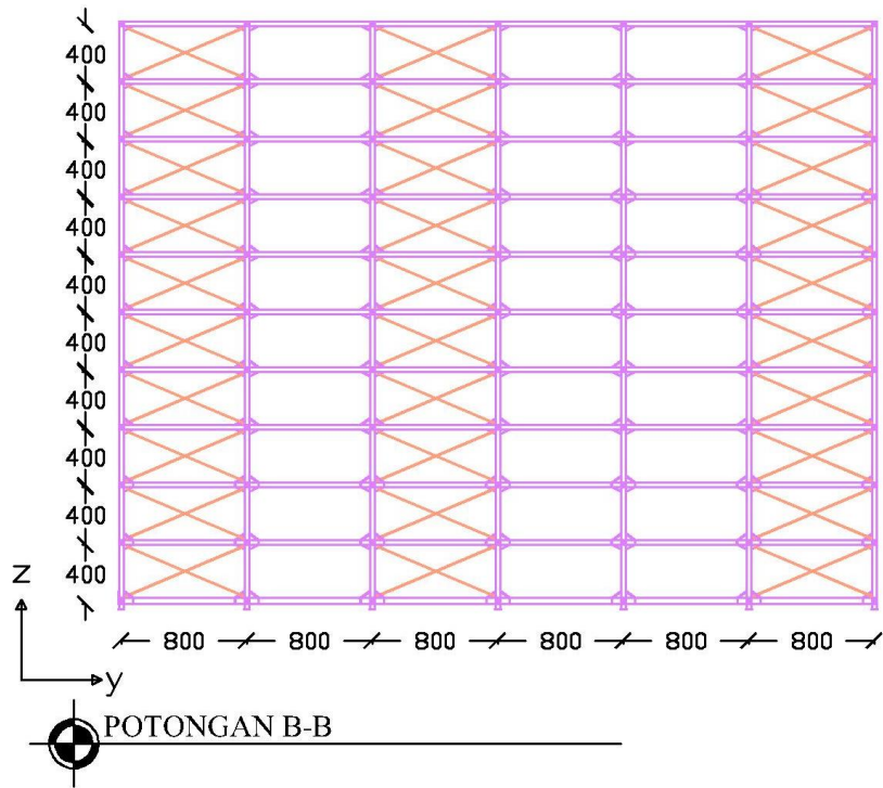
Gambar L-1.4 Potongan B-B Bangunan Bresing X 1-Lantai
