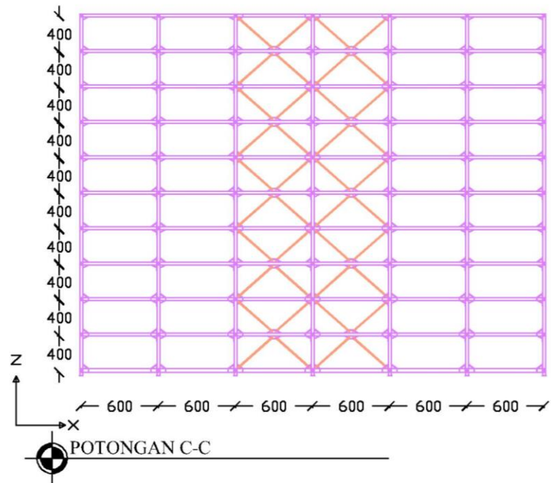
Gambar L-1.9 Potongan C-C Bangunan Bresing X 2-Lantai
