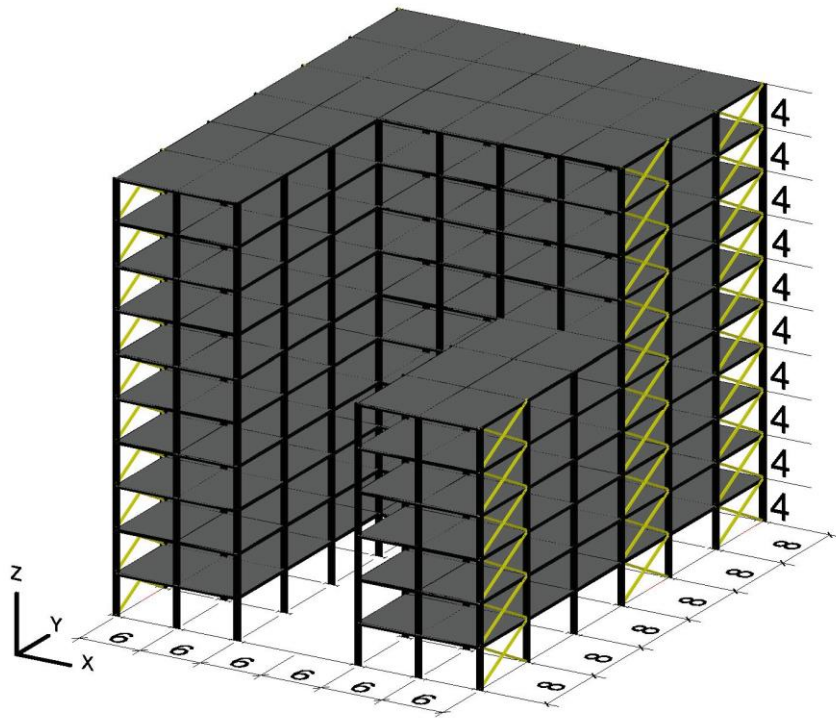
Gambar L-1.6 Pemodelan 3D Bangunan Bresing X 1-Story
