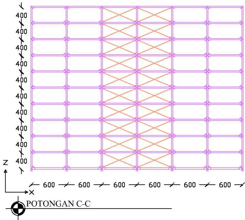
Gambar L-1.5 Potongan C-C Bangunan Bresing X 1-Lantai
