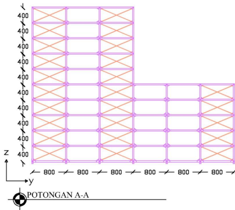
Gambar L-1.3 Potongan A-A Bangunan Bresing X 1-Lantai
