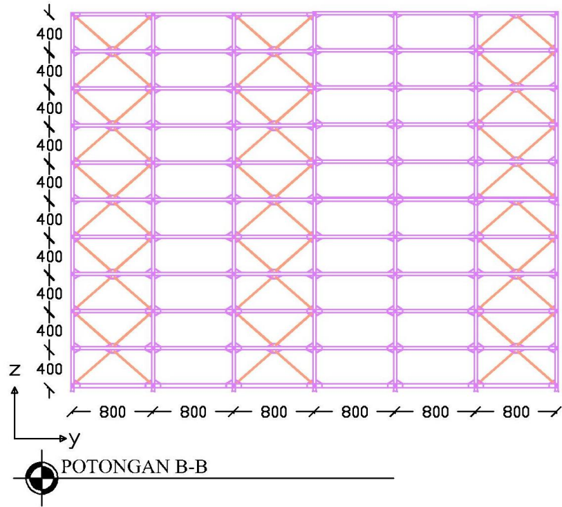
Gambar L-1.8 Potongan B-B Bangunan Bresing X 2-Lantai
