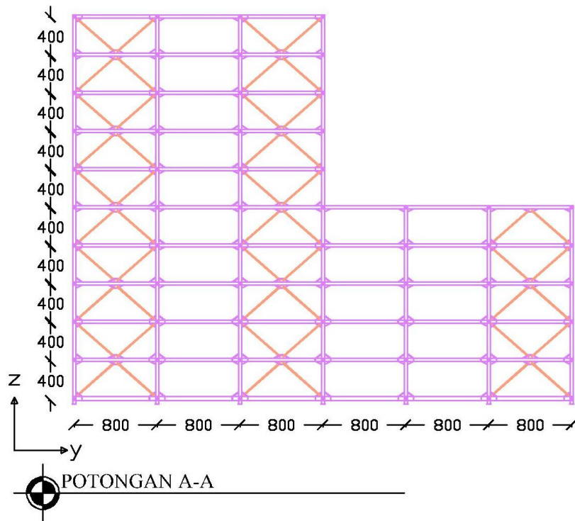
Gambar L-1.7 Potongan A-A Bangunan Bresing X 2-Lantai
