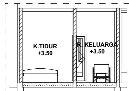
TIPE A 24 m2
