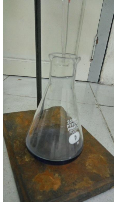
Pengujian BOD
