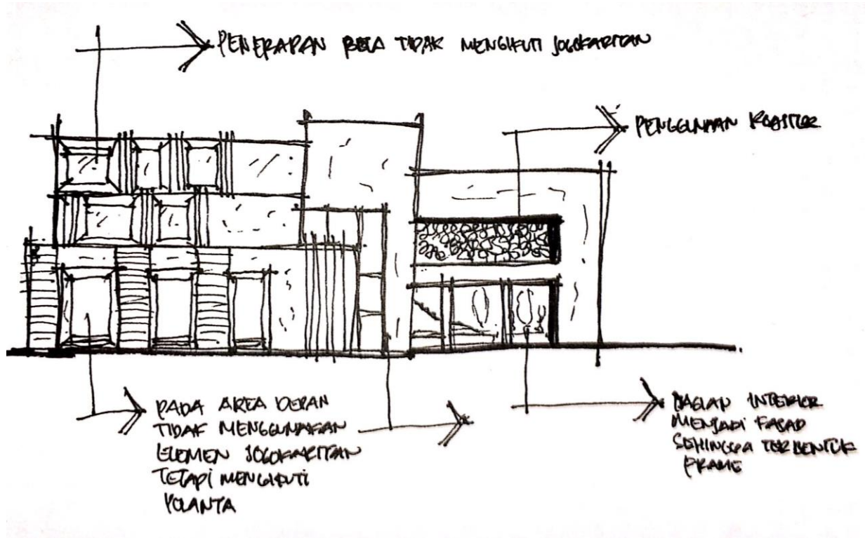
Gambar 4.7 Konesp fasad
