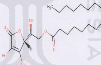
Gambar 2.5. Struktur kimia ascorbyl palmitate (6) .
