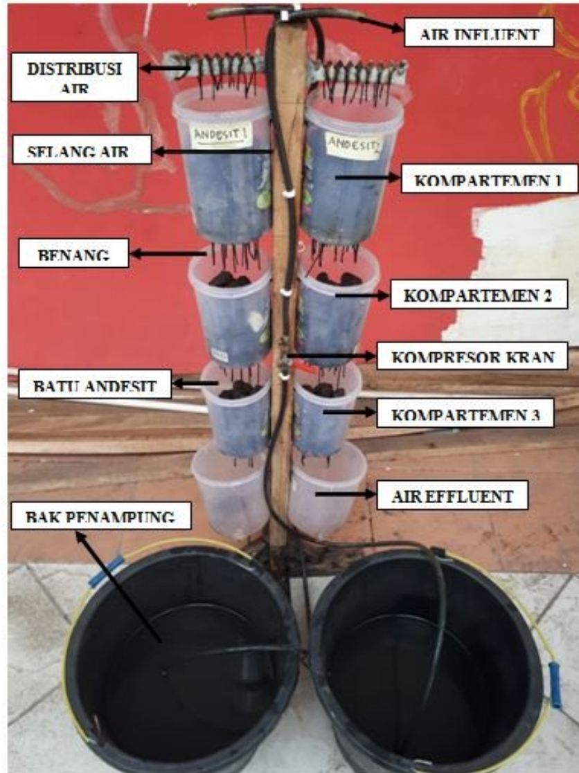
Lampiran 1. Gambar Tray Bioreactor dengan Media Batu Andesit
