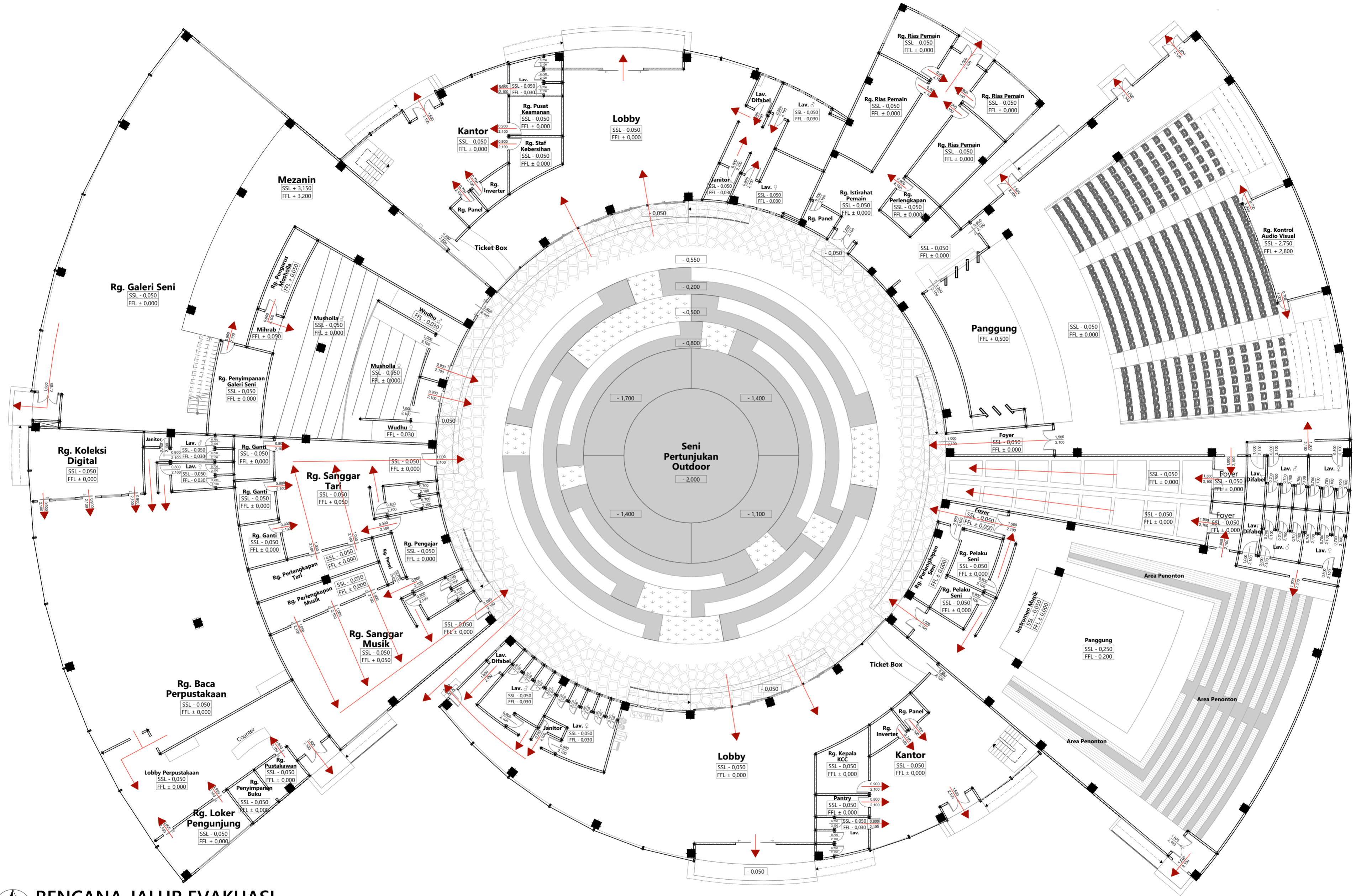
RENCANA JALUR EVAKUASI SKALA 1 : 200
