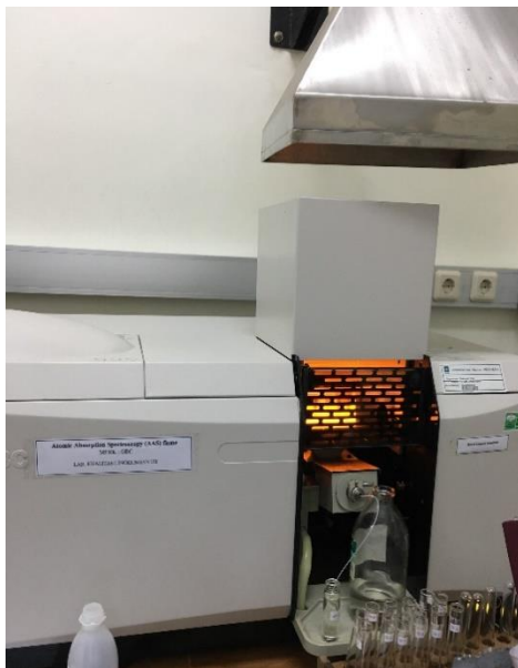
Gambar 3. Spektrofotometer Serapan Atom-Nyala
