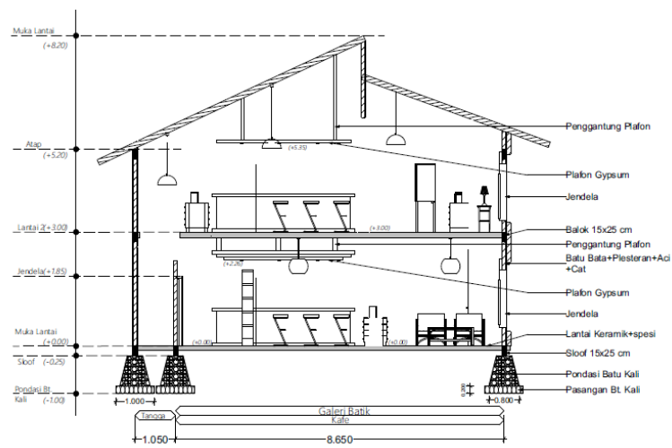
Gambar 6. 10 Potongan Bangunan Kafe dan Galeri Batik
