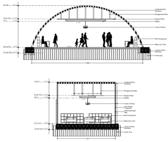
Gambar 6. 7 Potongan Bangunan Hall Sumber : Penulis, 2018
