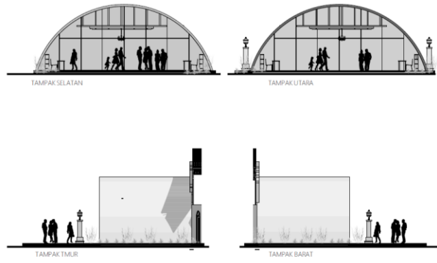
Gambar 6. 6 Tampak Bangunan Hall Sumber : Penulis, 2018
