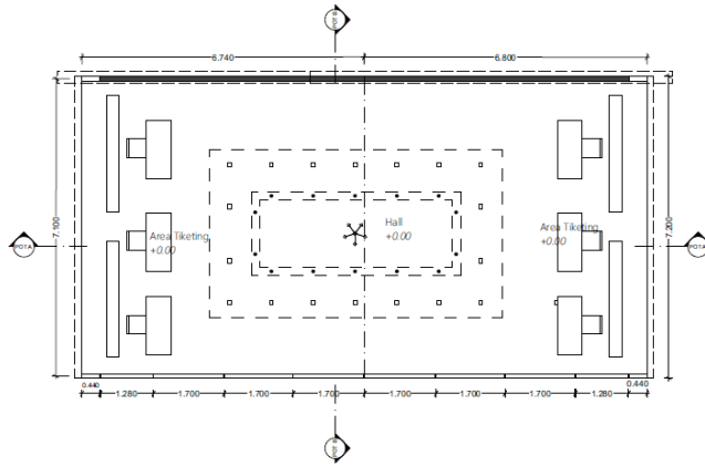
Gambar 6. 5 Denah Hall Sumber : Penulis, 2018
