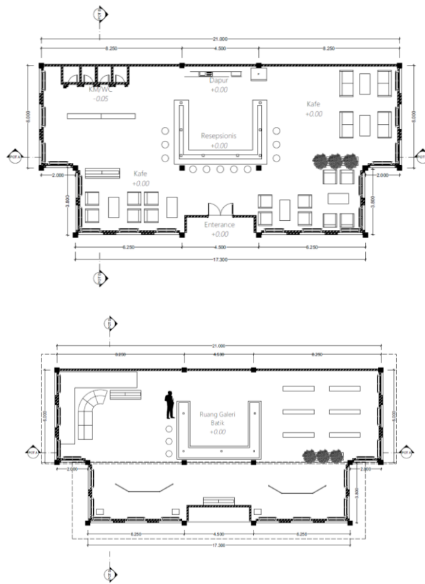
Gambar 6. 8 Denah Lantai 1 dan 2 Kafe dan Galeri Batik Sumber : Penulis, 2018
