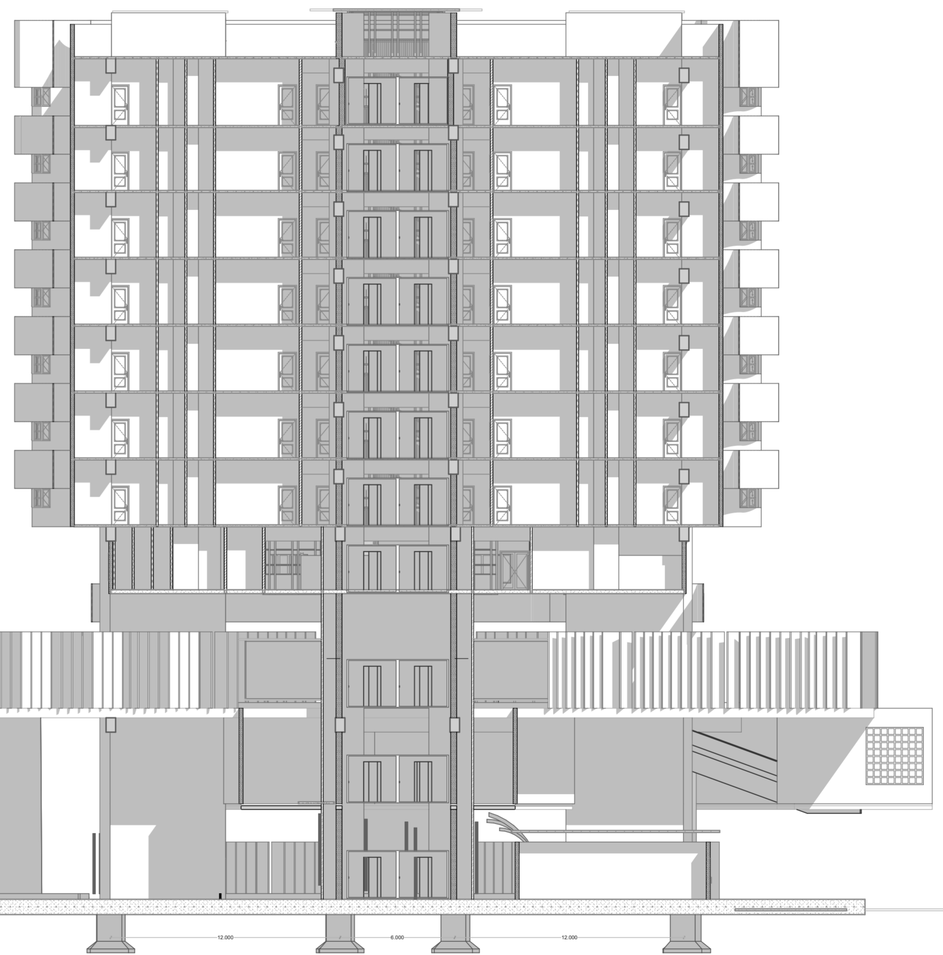
POTONGAN BB'
