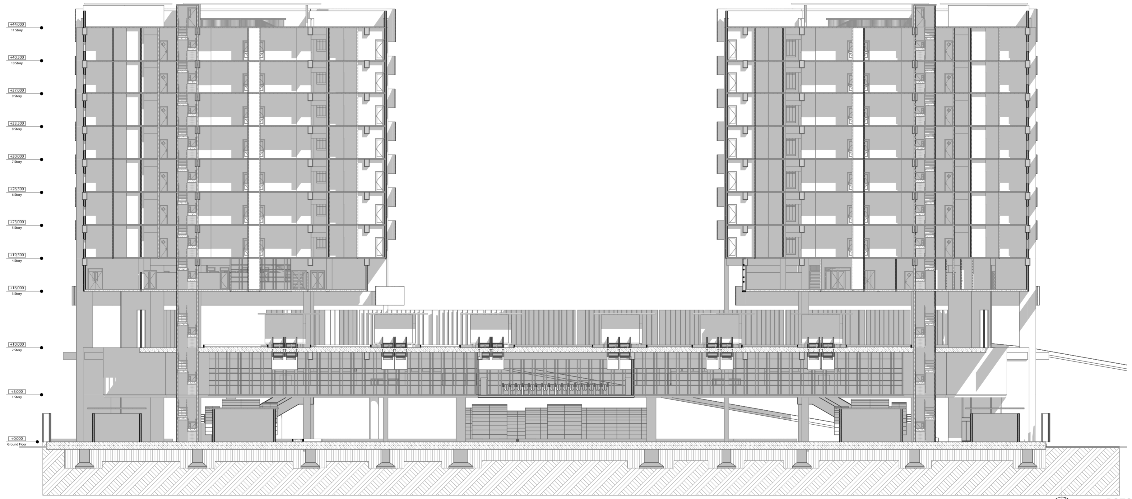
POTONGAN CC'
