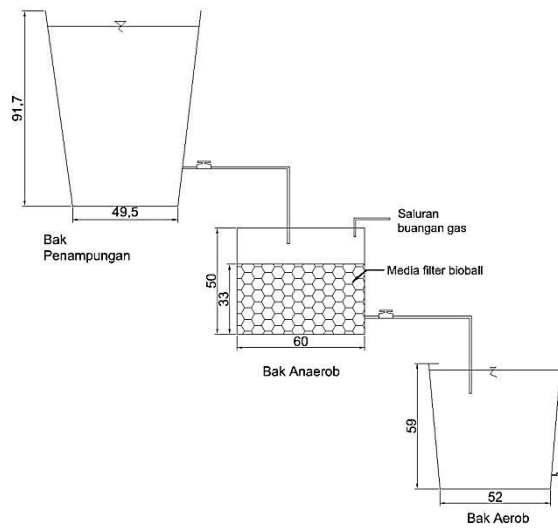
Desai Reaktor Kombinasi Anaerob-Aerob
