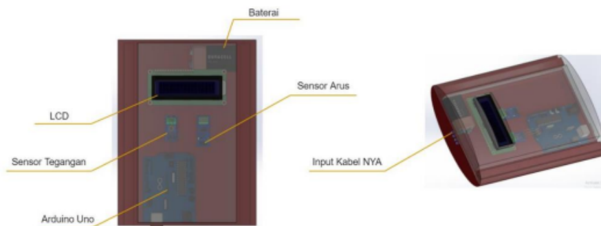
Gambar 1. Desain alat
