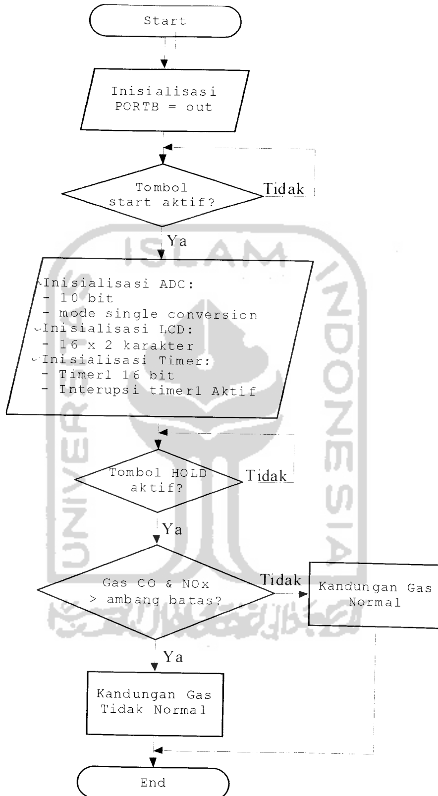
Gambar 3.12. Diagram alir program utama mikrokontroler.
