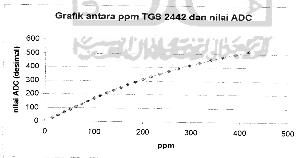
Gambar 4.9. Grafik pengujian ppm terhadap nilai ADC
