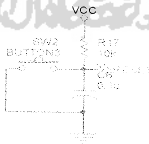
Gambar 3.6. Rangkaian reset
