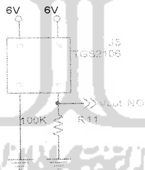
Gambar 3.3. Rangkaian sensor gas TGS 2106
