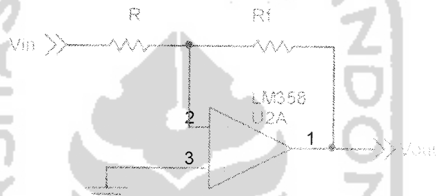
Gambar 2.7. Rangkaian penguat inverting
