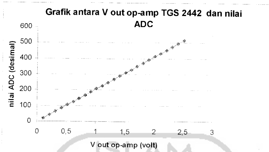
Gambar 4.5. Grafik pengujian V out op-amp TGS 2442 terhadap nilai ADC
