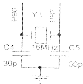
Gambar 3.5. Rangkaian osilator
