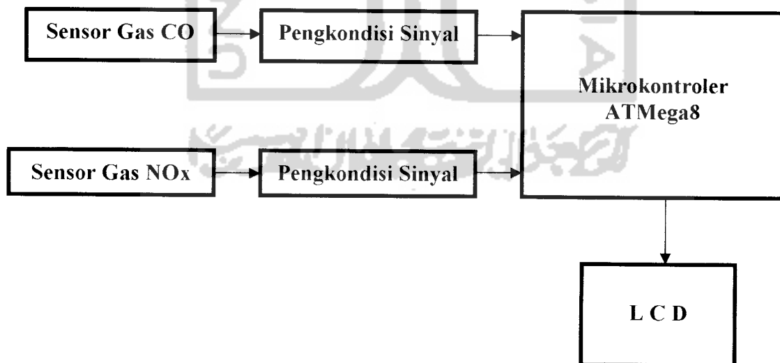
Gambar 3.1. Blok diagram keseluruhan sistem
