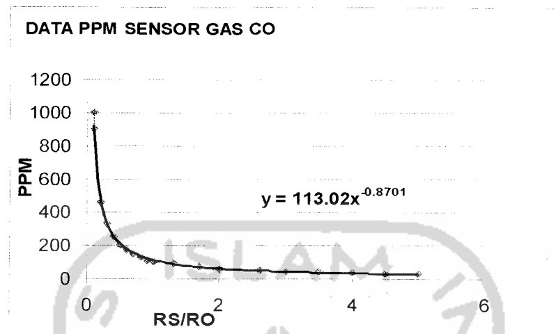
Gambar 4.7. Grafik hubungan nilai Rs/Ro terhadap ppm gas CO
