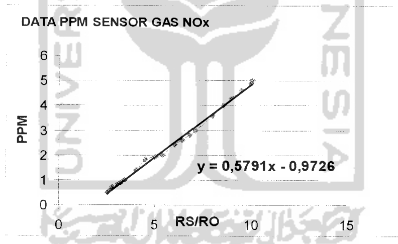
Gambar 4.8. Grafik hubungan nilai Rs/Ro terhadap ppm gas NOx
