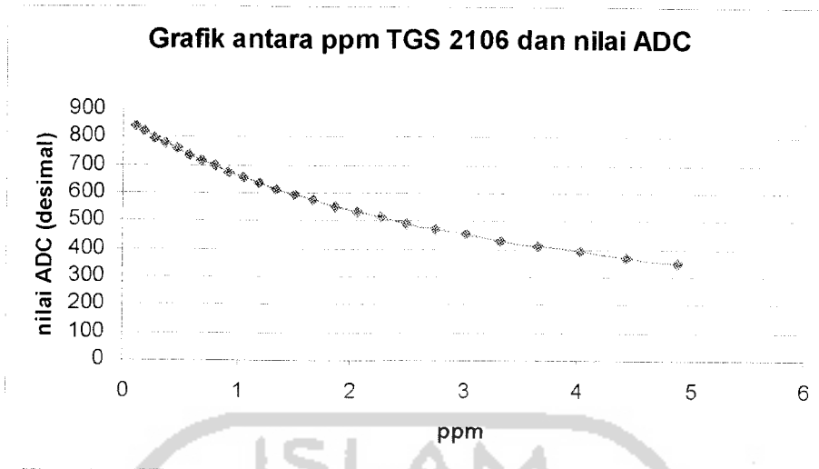
Gambar 4.10. Grafik pengujian ppm terhadap nilai ADC
