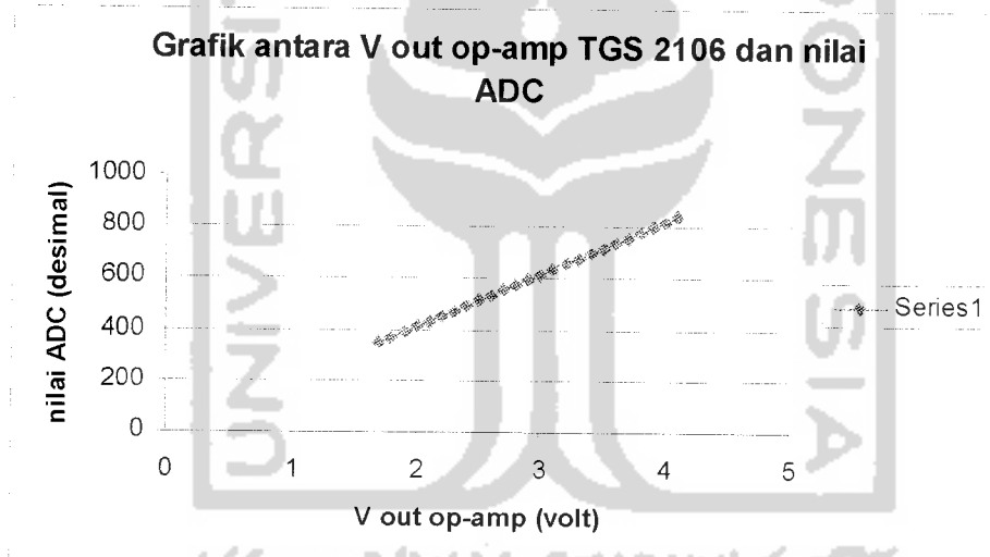
Gambar 4.6. Grafik pengujian V out op-amp TGS 2106 terhadap nilai ADC
