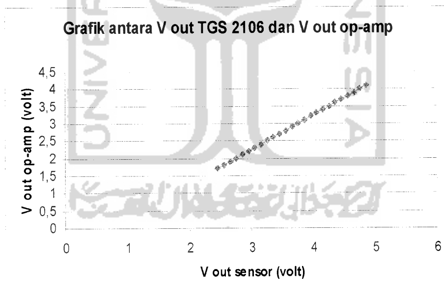
Gambar 4.3. Grafik pengukuran V out sensor TGS 2106 terhadap V out op-amp
