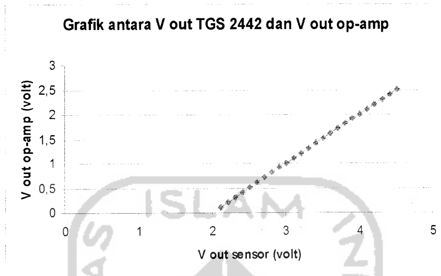
Gambar 4.2. Grafik pengukuran V out sensor TGS 2442 terhadap V out op-amp
