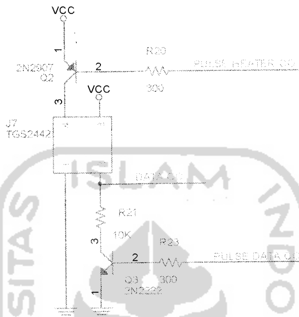
Gambar 3.2. Rangkaian sensor gas TGS 2442
