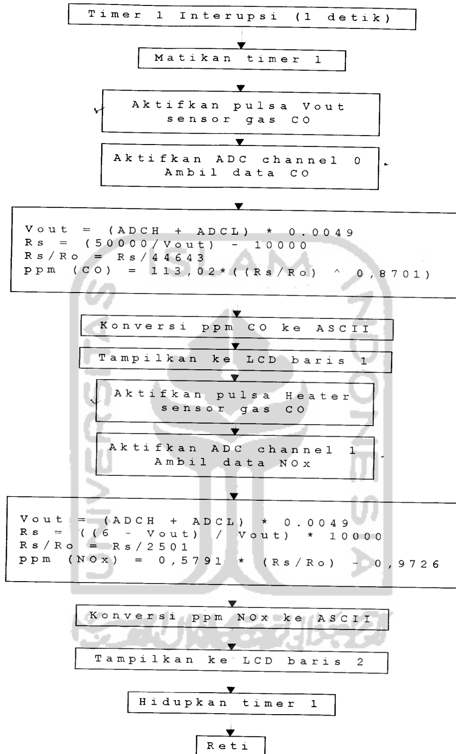
Gambar 3.12. Diagram alir program timer, ADC dan konversi ppm ASCII.
