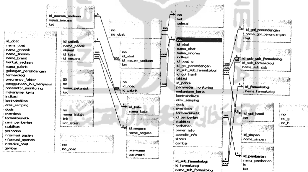
Gambar 3.8. Skema relasi antar tabel
