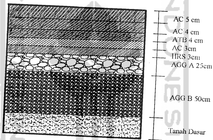
Gambar 5.25 Perencanaan Tebal Lapis Keras Tambahan ( Overlay )
