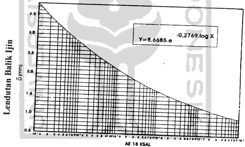
Gambar 3.8 Grafik Penentuan Nilai Defleksi yang Diijinkan
