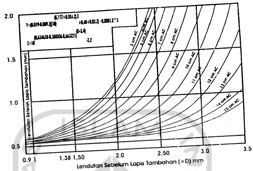
Gambar 3.9. Grafik Penentuan Tebal Overlay Metode Bina Marga 1983 Sumber : Bina Marga, 1983
