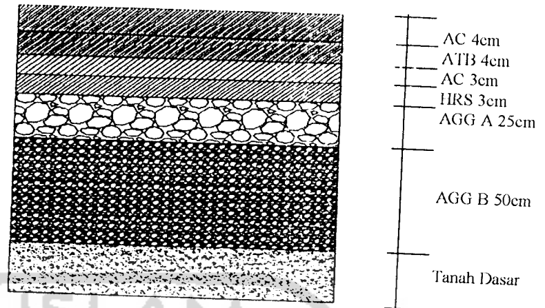
Gambar 5.9 Struktur Perkerasan Jalan Magelang-Keprakan Sumber : Sub Dinas Bina Marga Propinsi Jawa Tengah
