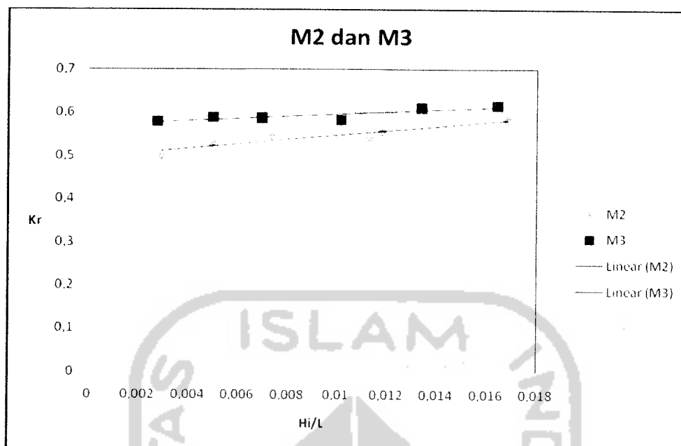
Gambar 6.2 Hubungan K_r dan H_i/L untuk model M2 dan M3
