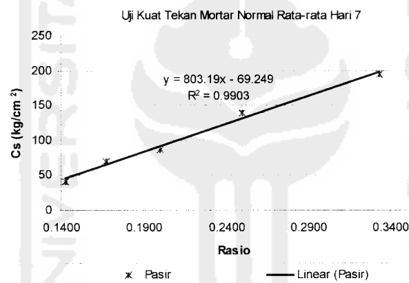
Gambar 5.2 Regresi uji kuat tekan mortar normal rata-rata umur 7 hari
