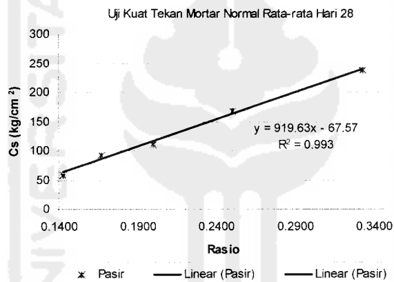
Gambar 5.5 Regresi uji kuat tekan mortar normal rata-rata umur 28 hari
