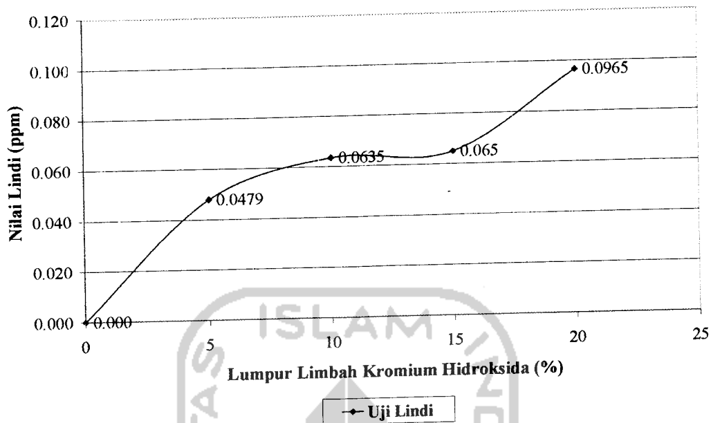
Gambar I.12 Grafik korelasi antara nilai lindi terhadap lumpur limbah kromium hidroksida pada suhu 1000°C.
