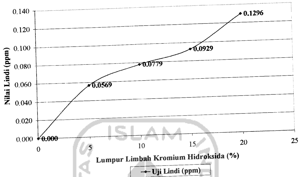
Gambar I.4 Grafik korelasi antara nilai lindi terhadap lumpur limbah kromium hidroksida pada suhu 800°C.
